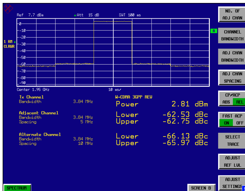
Bild 2.37 Messung der Nachbarkanalleistung eines W-CDMA-Signals mit der Fast-ACP-Methode.
