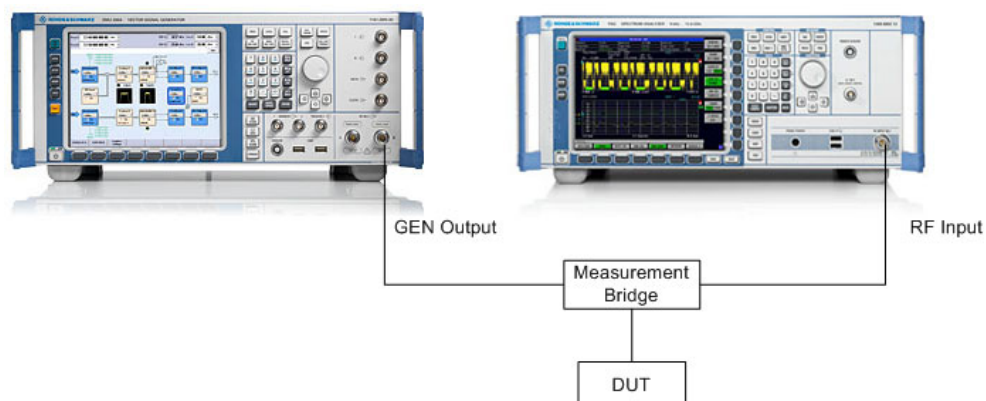
Bild 4.38 Anordnung für Reflexionsmessungen
