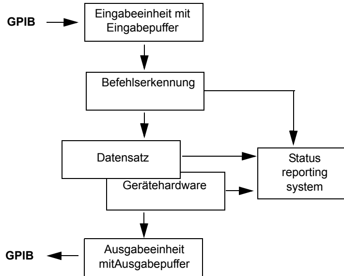
Bild 5.11 Gerätemodell bei Fernsteuerung
