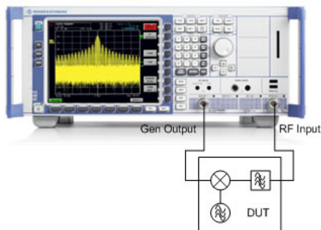
Bild 4.30 Anordnung für frequenzumsetzende Messungen
