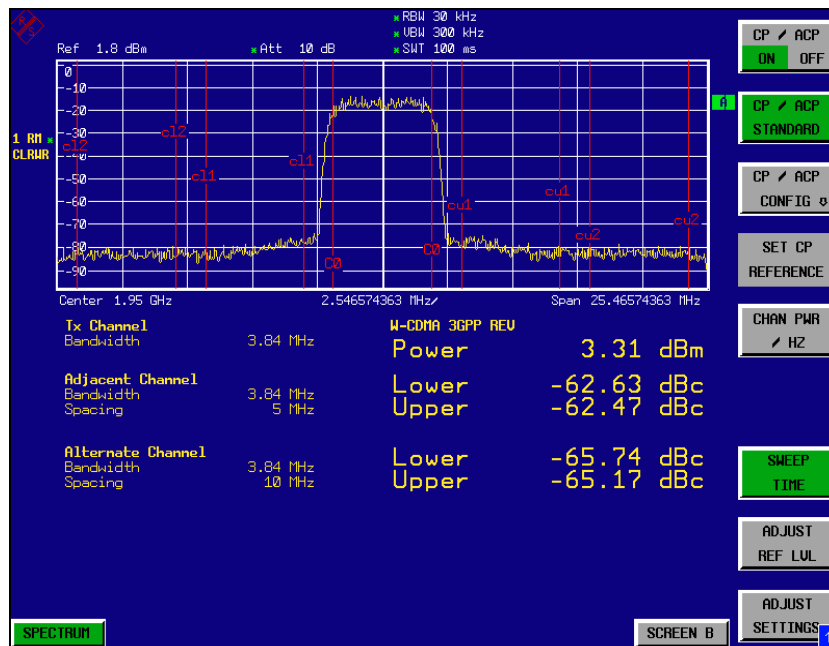
Bild 2.36 Messung der relativen Nachbarkanalleistung an einem W-CDMA-Uplink-Signal.
