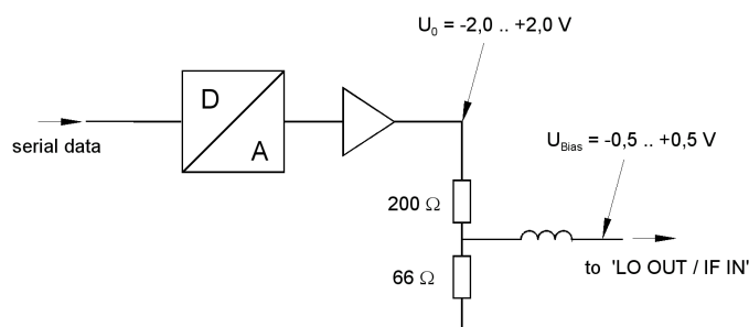
Bild 4.40 Bias-Schaltung des R&S FSU
