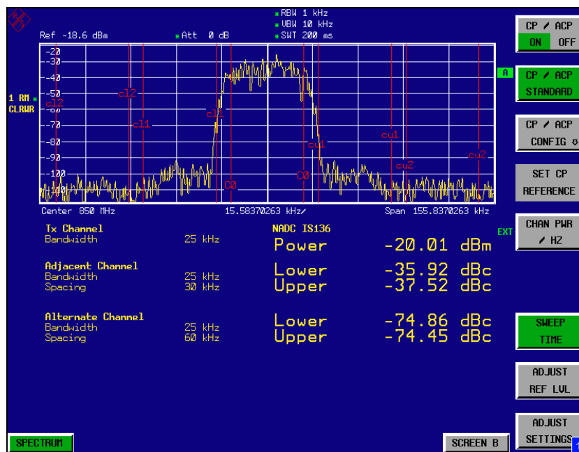
Bild 2.31 Messung der relativen Nachbarkanalleistung eines NADC-Signals in je zwei Nachbarkanälen unterhalb und oberhalb des Sendekanals.
