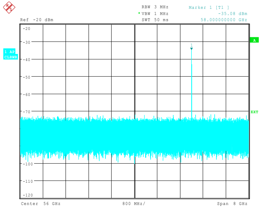
Bild 4.46 Ausgangsspektrum des Vervielfachers aufgenommen mit Hilfe eines externen Mischers und AUTO ID
