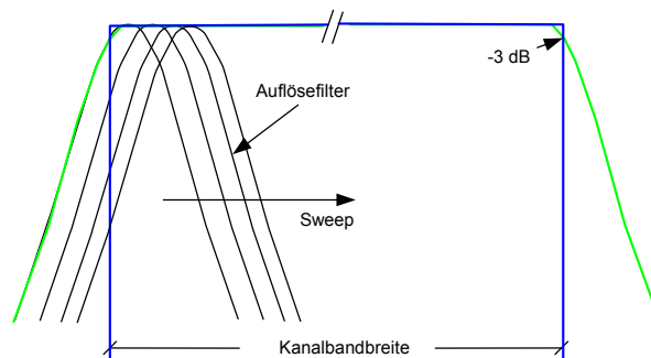
Bild 2.18 Approximation des Kanalfilters durch Sweeps mit kleiner Auflösesebandbreite
